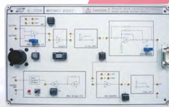
體阻抗測量模組 (裝有心律調整器者嚴禁使用此實驗)
