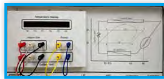
系統和電氣連接 實踐中的溫度點、 莫里爾圖
